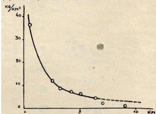
Fig. 3. Wykres „nasilenia” meteoritów (w kg. na km 2 ) na obszarze ich spadku (w km bieżących).
